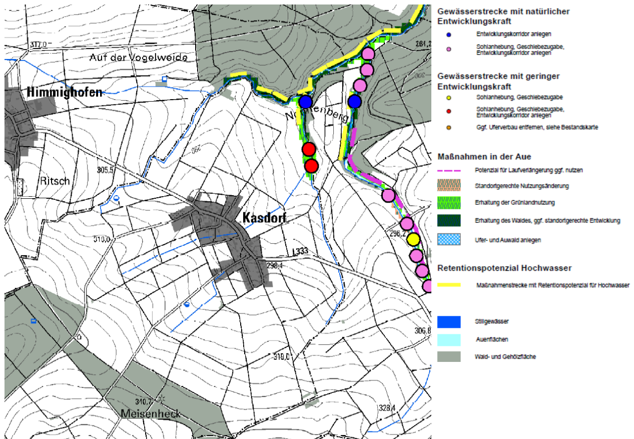
Abbildung 7: Maßnahmen an Gewässer und Aue, Karte 2 (LfU, 2020)
