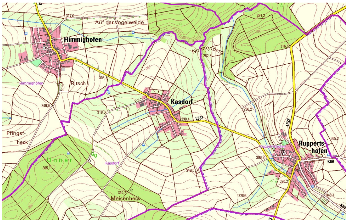
Abbildung 5: Topographische Gegebenheiten der Ortsgemeinde Kasdorf (Quelle: LANIS, 2024)
