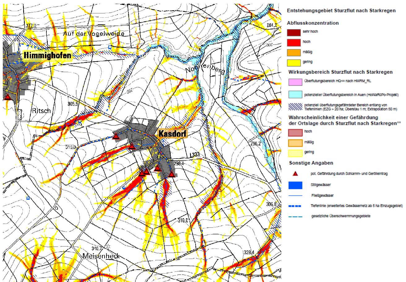
Abbildung 10: Gefährdungsanalyse Sturzflut nach Starkregen, Karte 5 (LfU, 2020)
