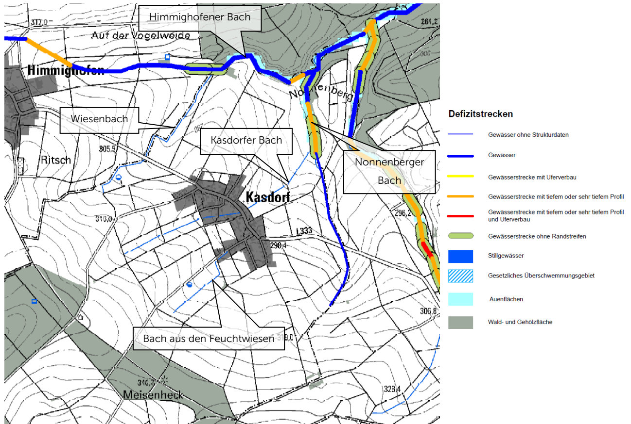
Abbildung 6: Bestand Gewässer und Aue Ortsgemeinde Kasdorf, Karte 1 (LfU, 2020)
